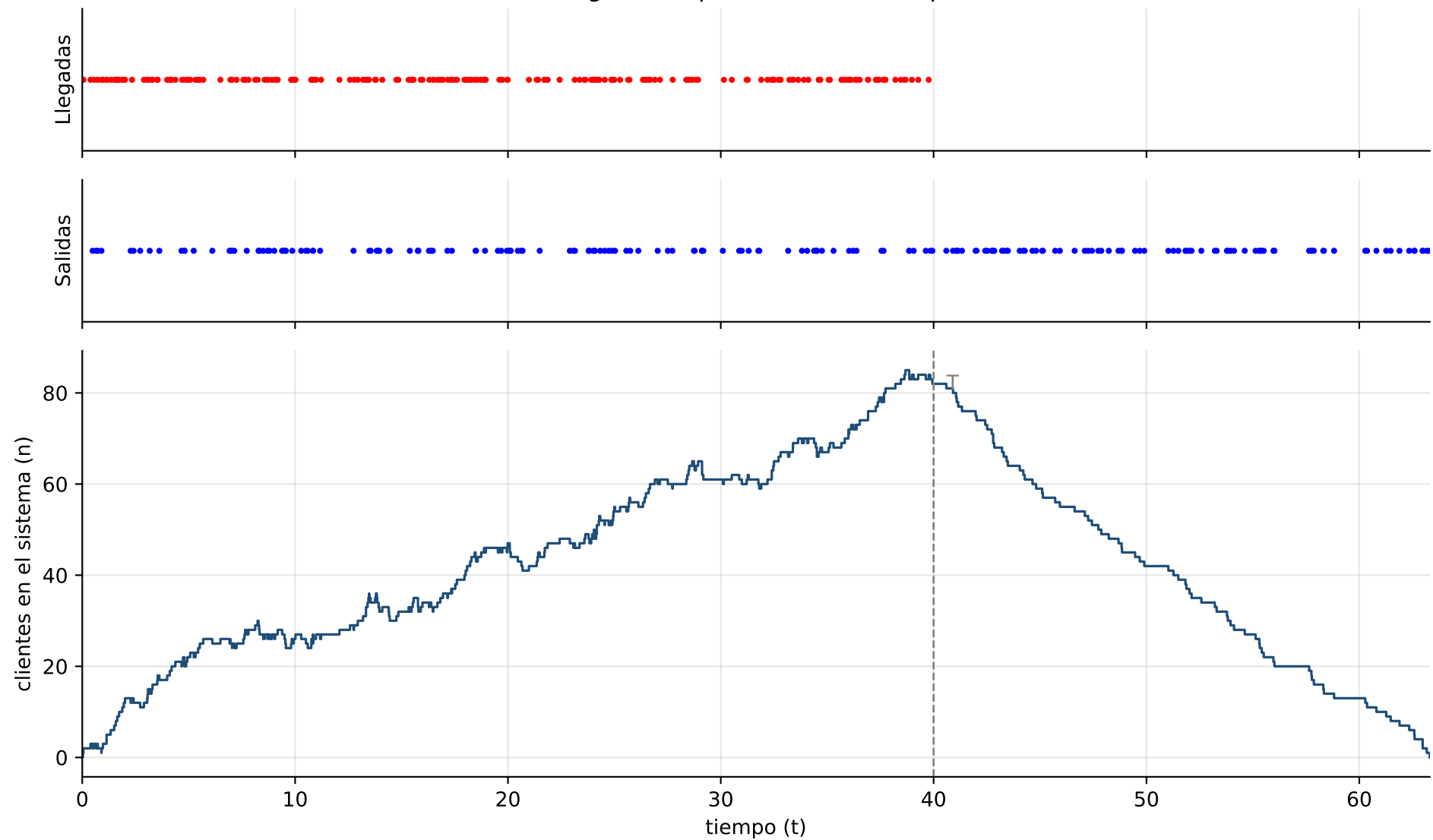
Escenario A: Llegadas Exp( \lambda=5 ), servicio Exp( \lambda=3 ), T = 40
